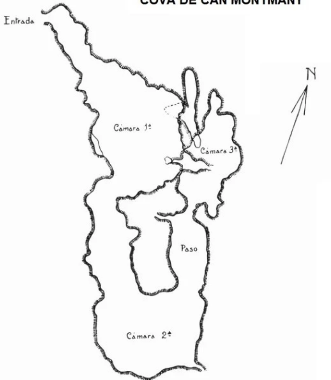
Fig. 1. — Plano de la cueva de Can Montmany, de Pallejà (Barcelona)
