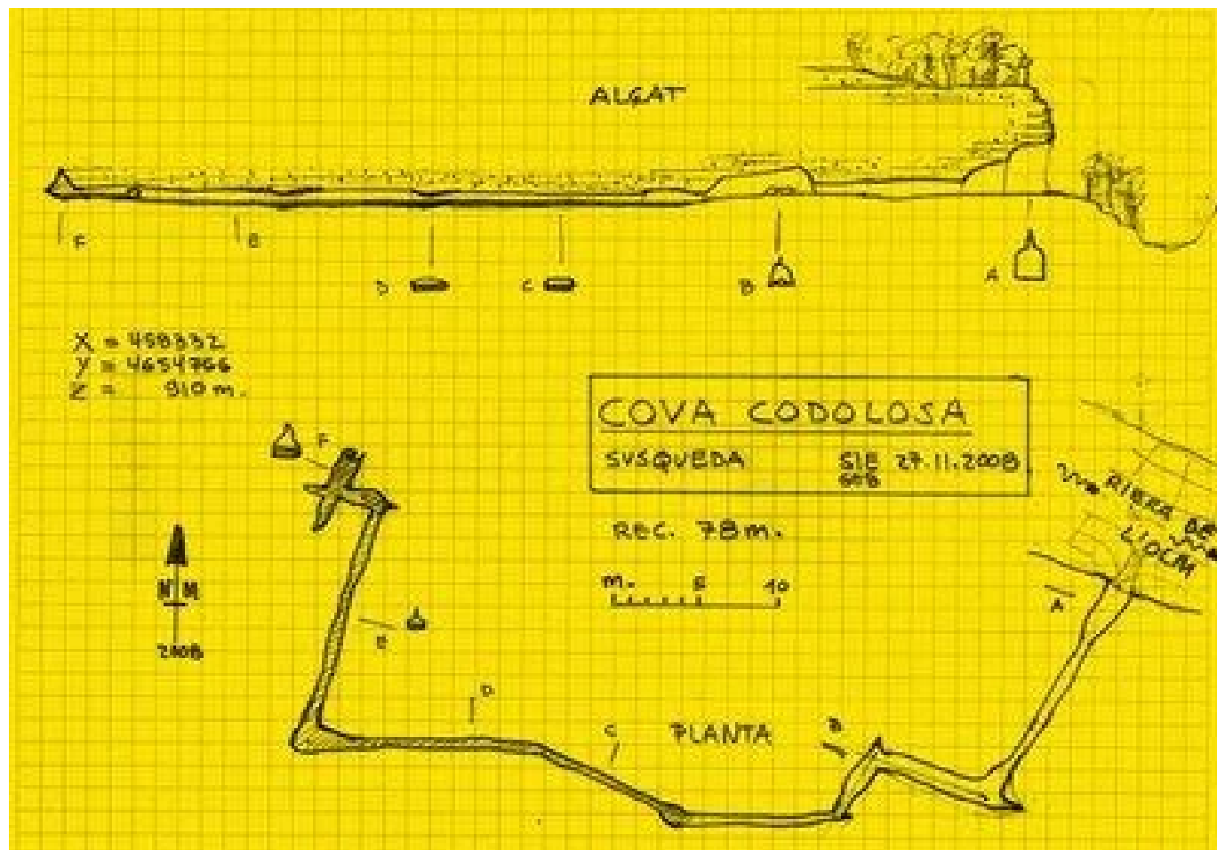
Topografia 2 de 2
