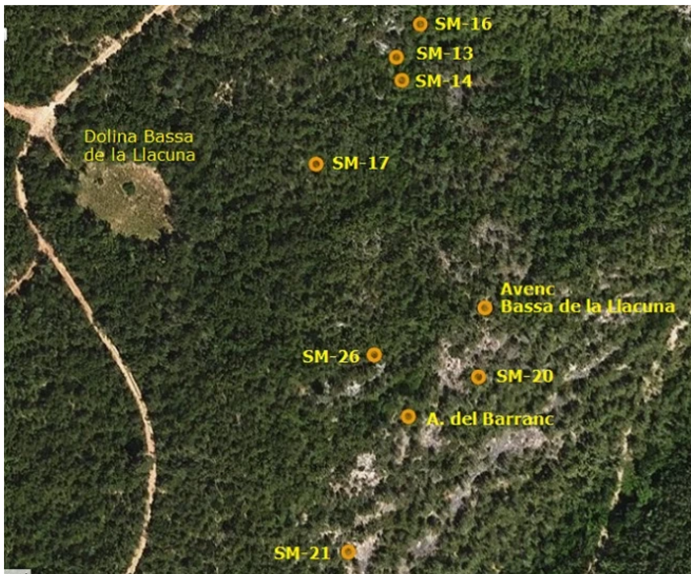
Topografia 1 de 2
