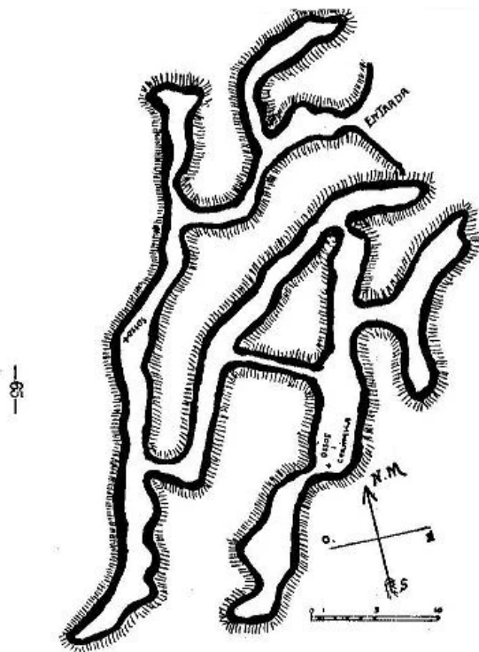
Cova Fonda de Salomé (Vilabella): Evolución de la topografía subterránea; comparación de los planos levantados en 1908 (F. Bertrán) y en 1934 (J. Closas). Obsérvese que únicamente en el segundo puede verse la estructuración sobre diaclasas (el plano de 1908, ha sido colocado al revés pues posee la orientación invertida.)
