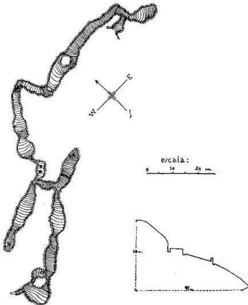
Representació plana de l'avenc de la Pòpia i desnivell del mateix (Joan Ferrate 17-7-1917)
