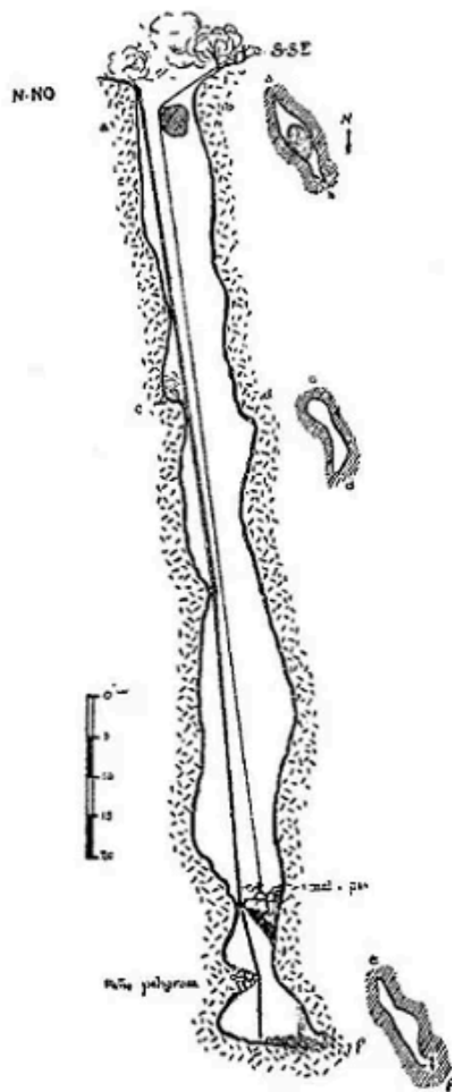
FIG. 18.—AVENCH DE LA COSTA-DRETA. Montserrat. Sección vertical (N.-NO. á S.-SE.) Profundidad, 120 metros.
