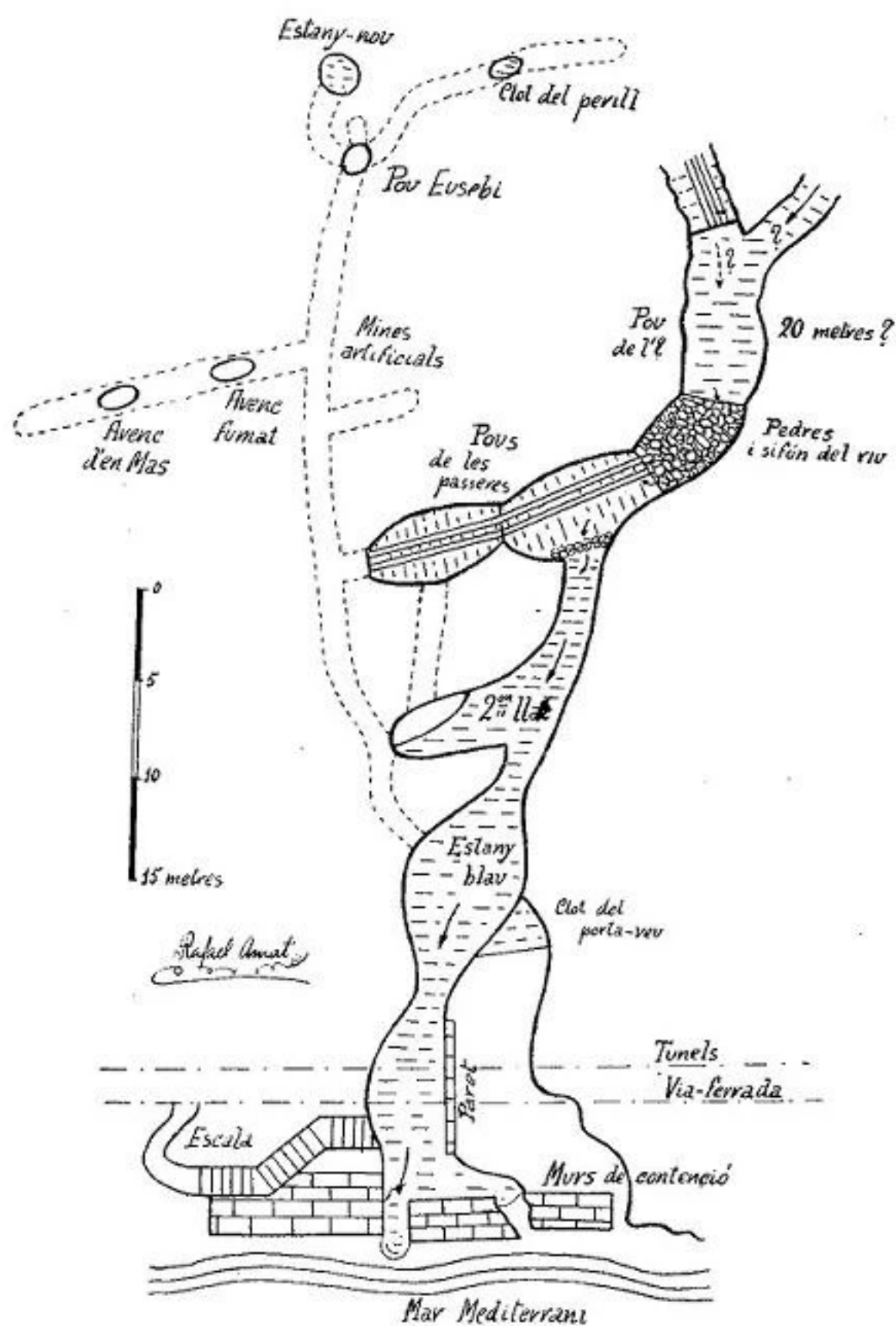
Planta de les coves de La Falconera .
