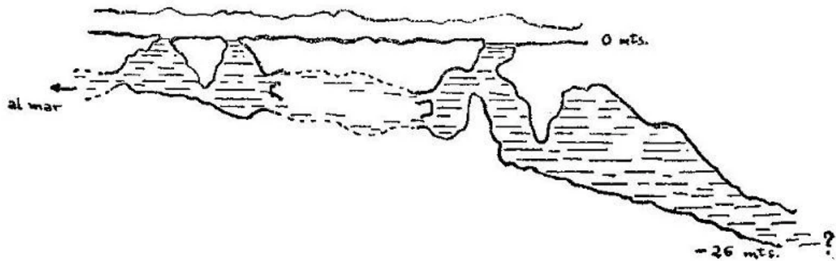
FIG. 12. — Secció longitudinal de la sorgència de La Falconera (Garraf).
