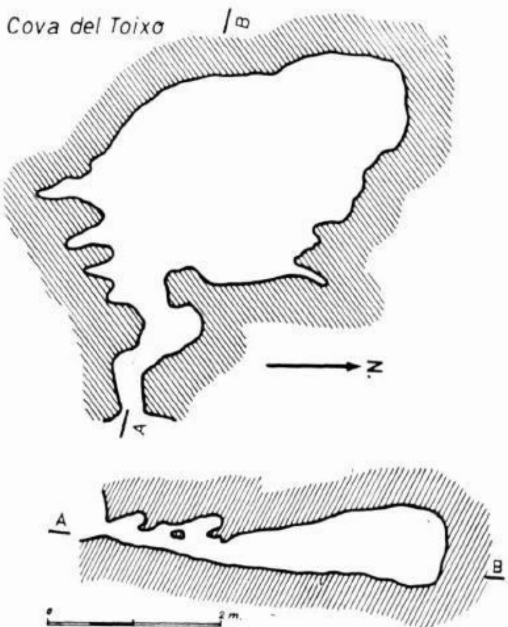
Fig. 37. — Planta y sección de la Cova del Toixó, en Torrelles de Foix.
