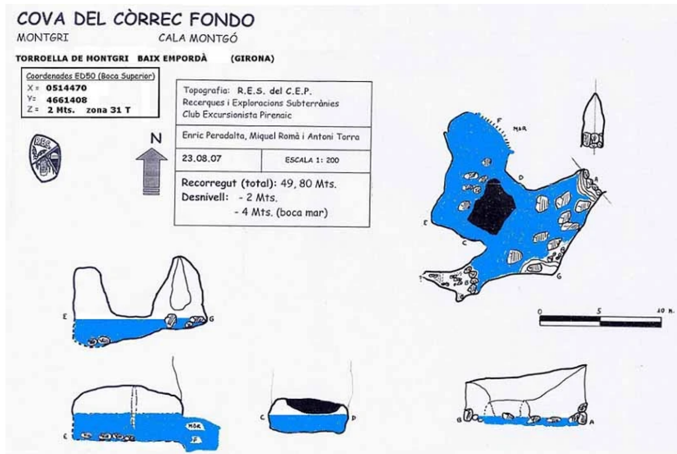
Topografia 1 de 1
