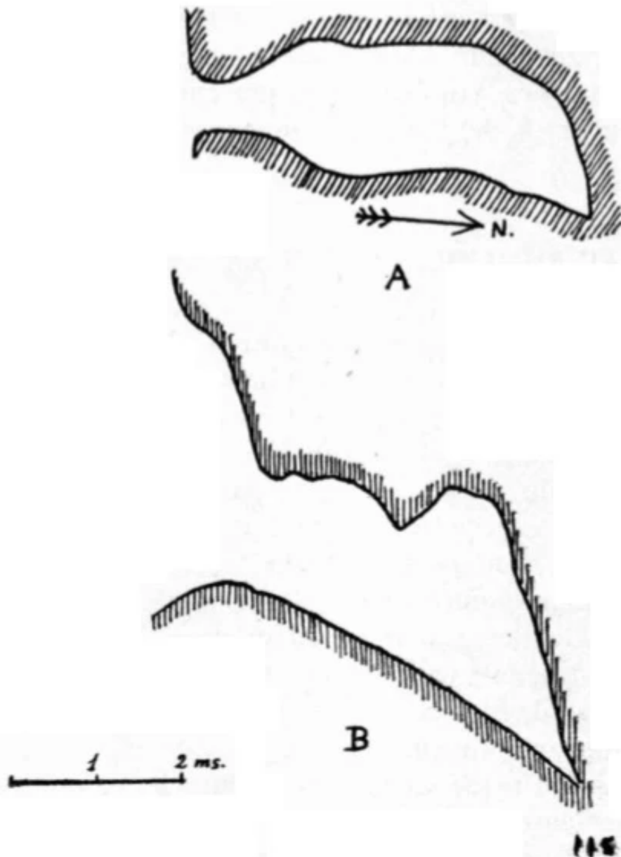
Croquis de la planta (A) y sección (B) del Cau de l'Olivar d'en Margall. (Torroella de Montgrí).
