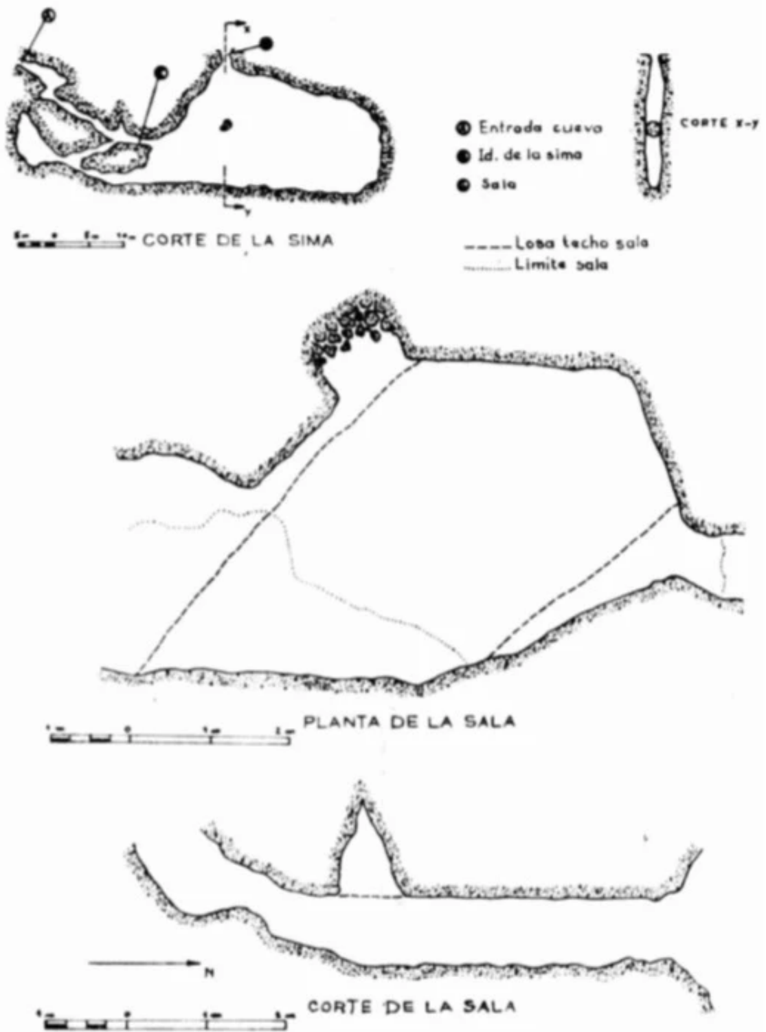
Fig. 4. — Planta y alzados de la Cueva del Daniel (Capafonts). (Dibujo de A. Gironés.)
