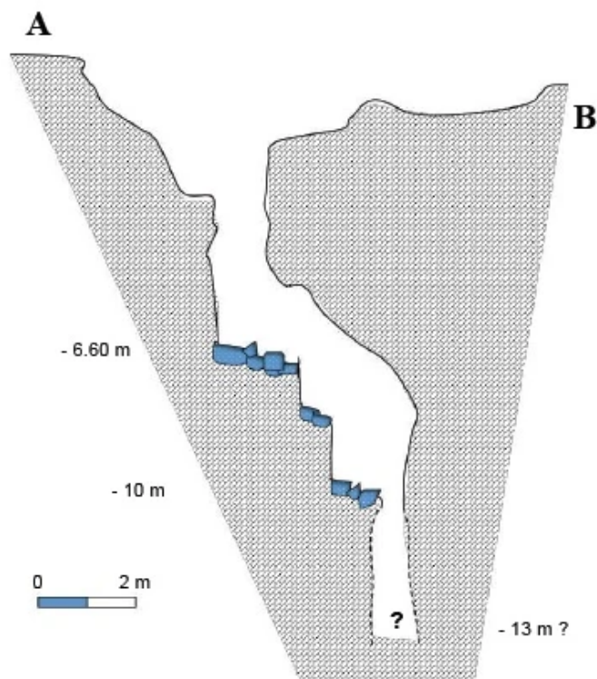
Coupe développée
