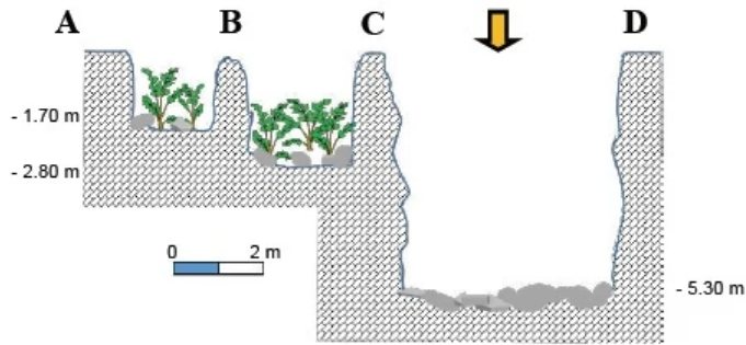
Coupe développée
