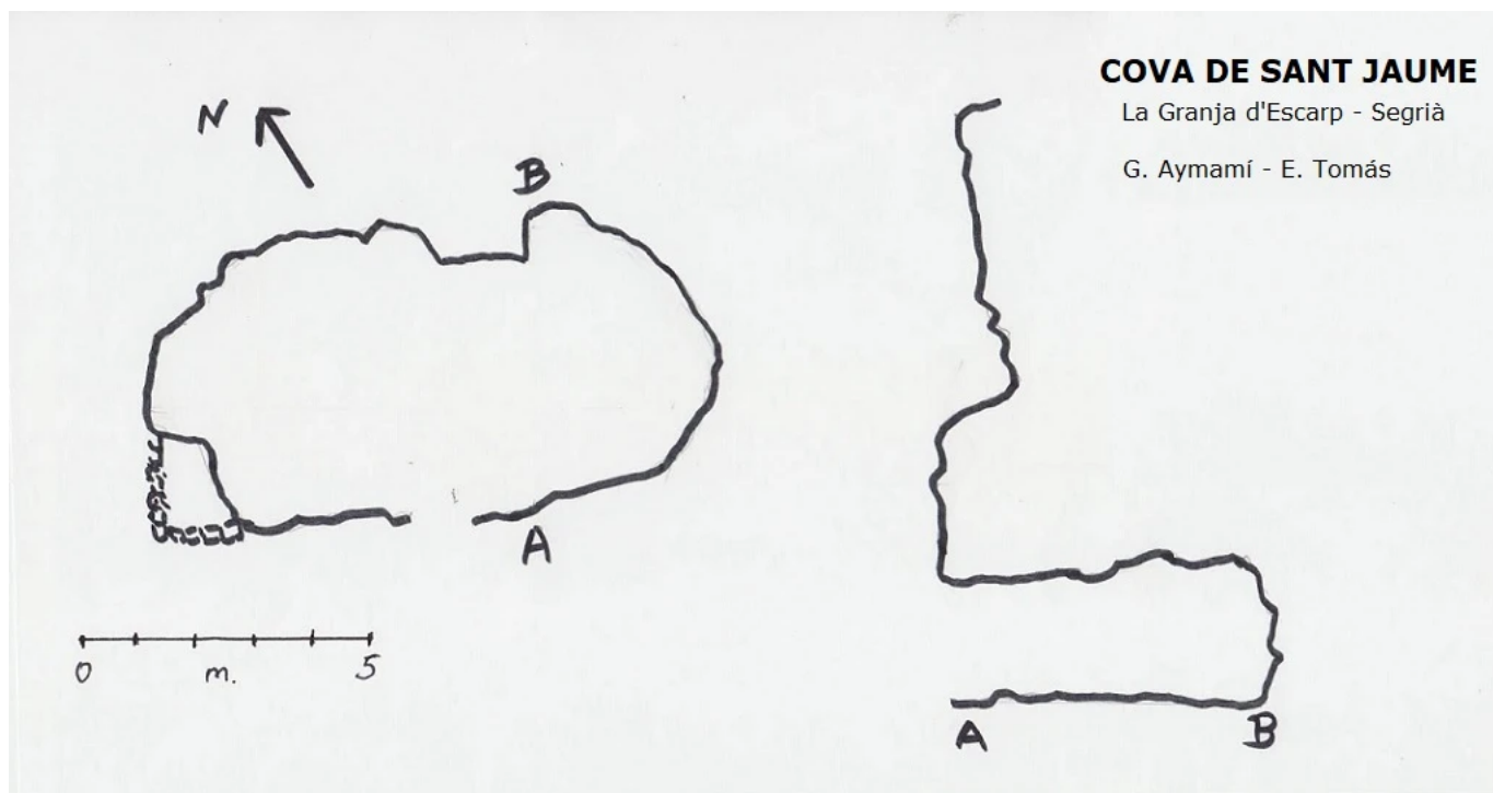
Topografia 1 de 1
